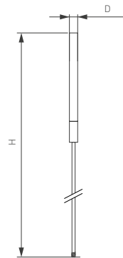
Рис. 1. Чертеж и габаритные размеры
