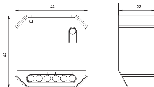
Рис. 1. Габаритные размеры
