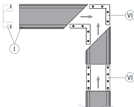
Рис. 1. Виды соединений
