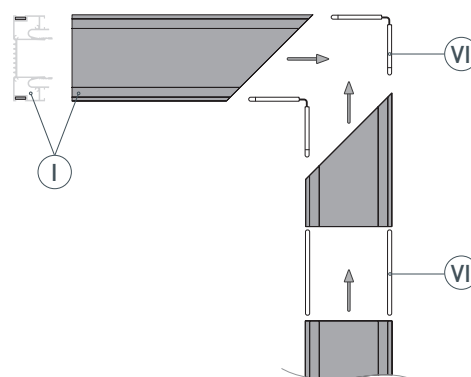
Рис. 2. Виды соединений
