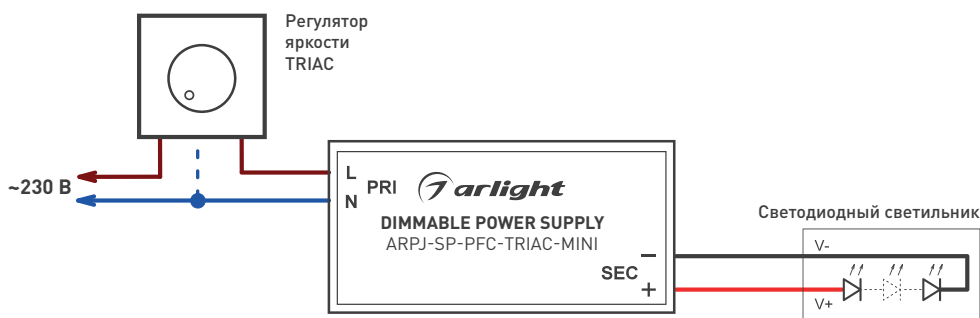
Рис. 1. Подключение драйвера.
