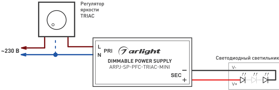
Рис. 1. Подключение драйвера.
